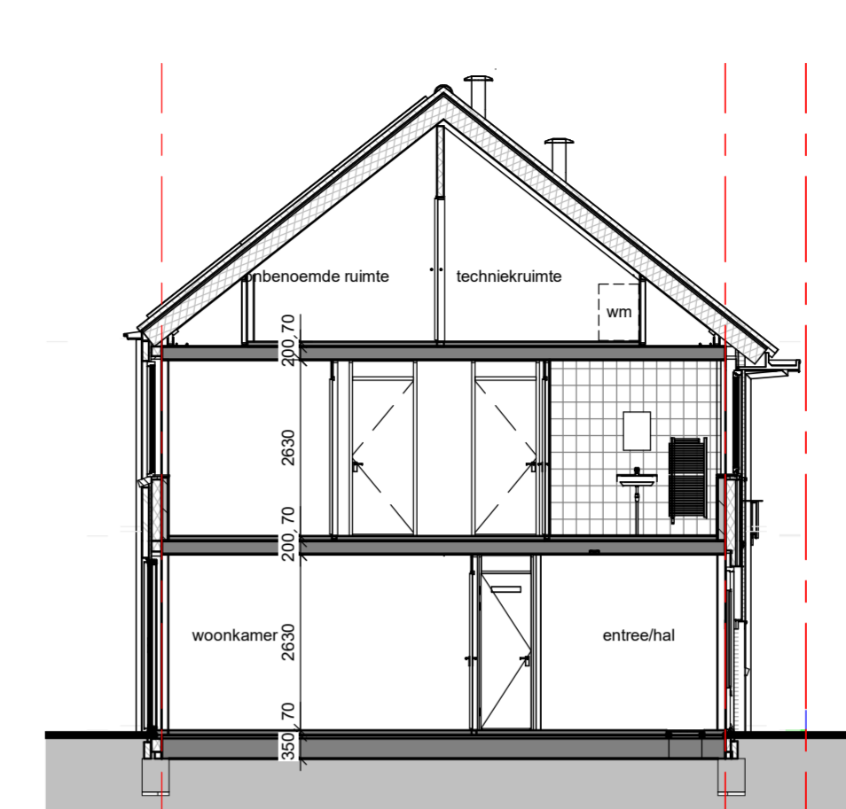
Doorsnede H-B
