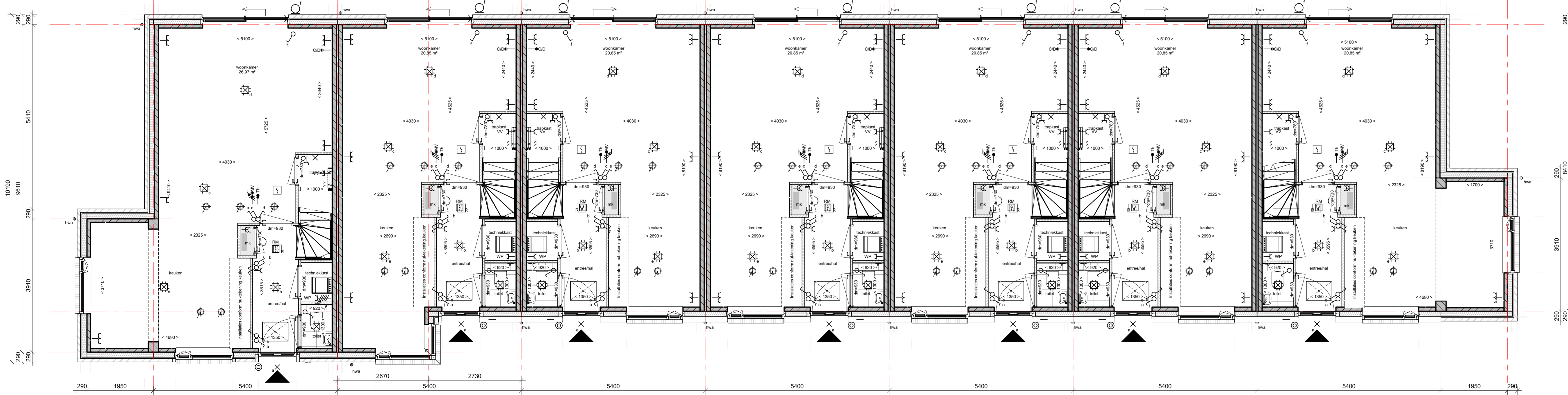
Begane grond Blok H
