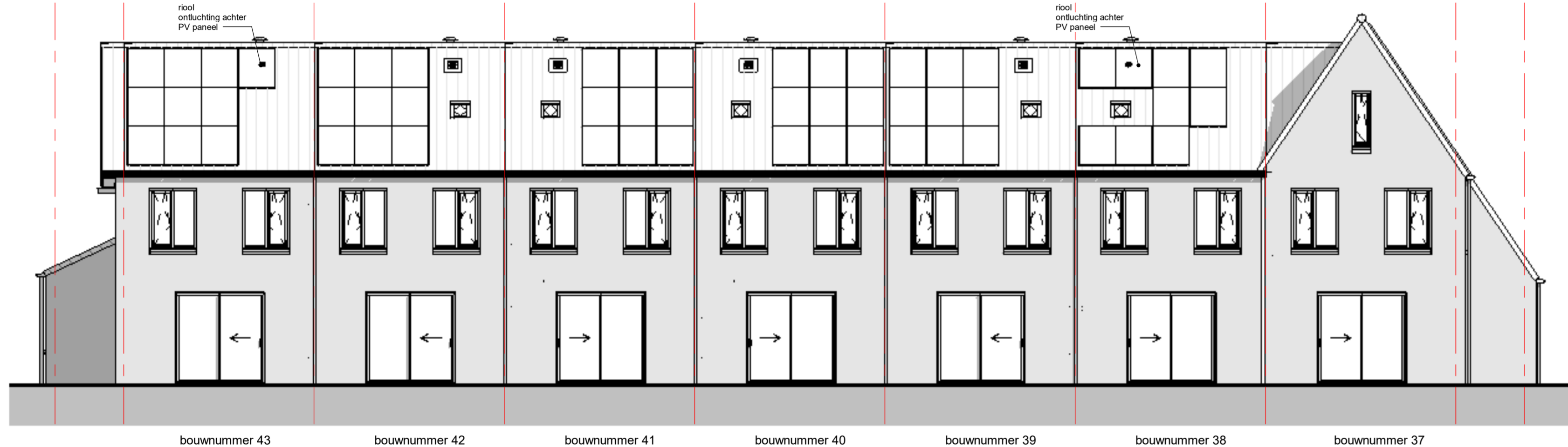
Achtergevel Blok H
