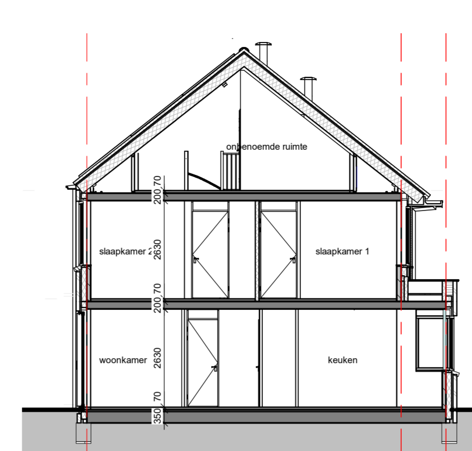
Doorsnede H-A
