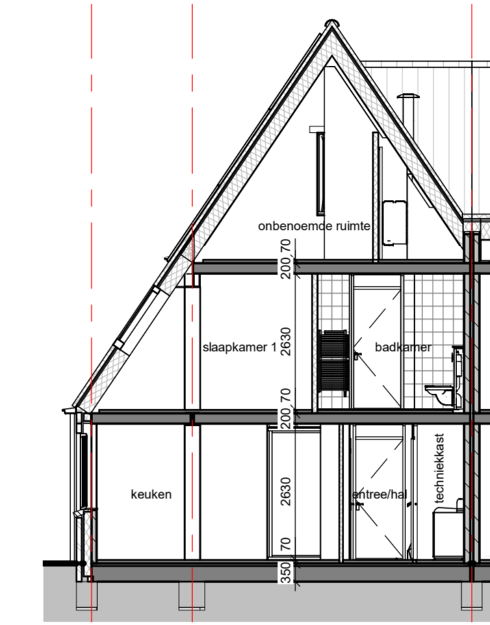
Doorsnede H-C
