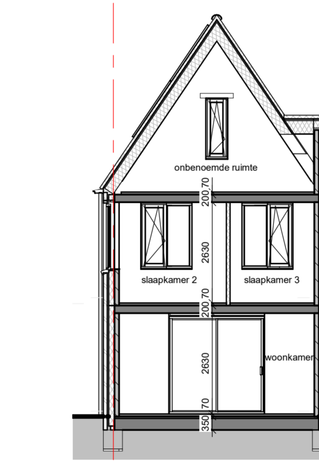
Doorsnede H-D
