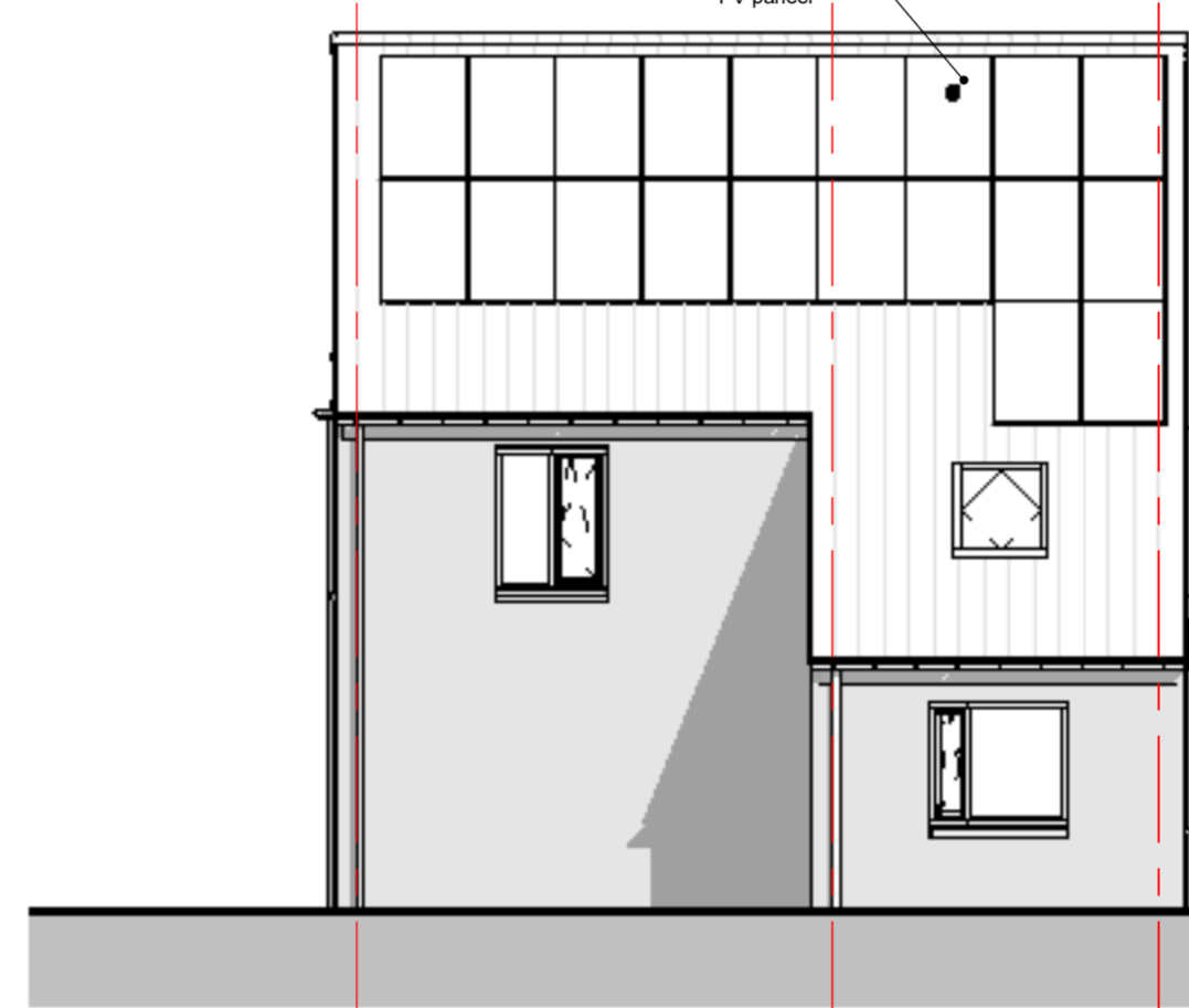
Linker zijgevel Blok H
