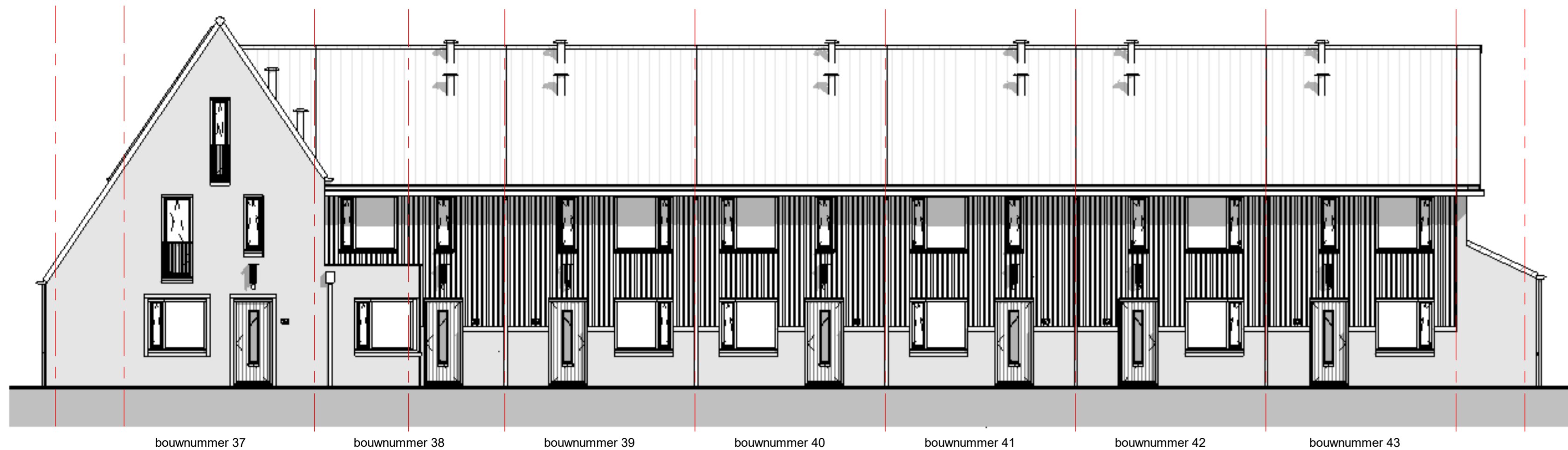
Voorgevel Blok H
