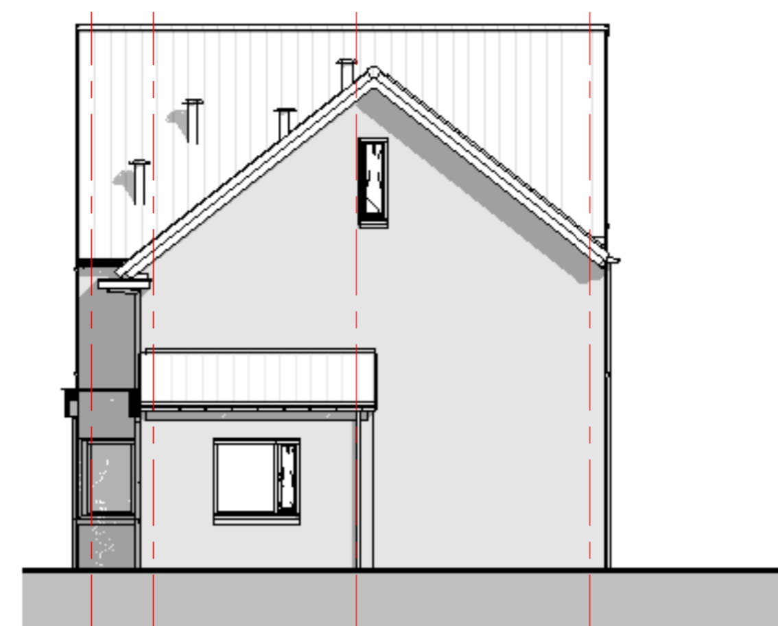
Rechter zijgevel Blok H
