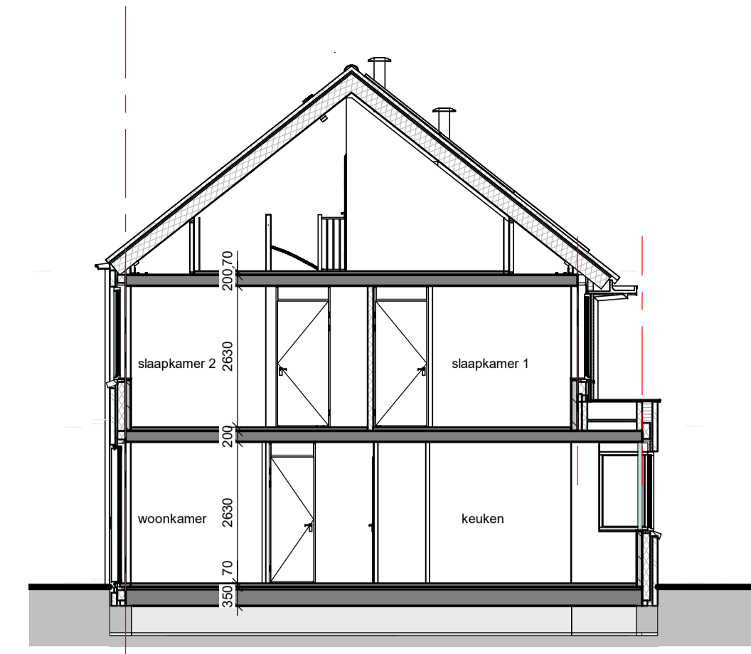
Doorsnede A-A schaal 1:100
