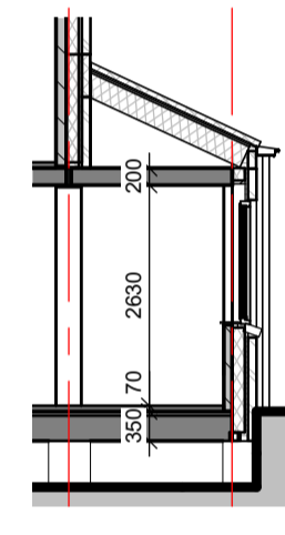
Doorsnede A-E schaal 1:100
