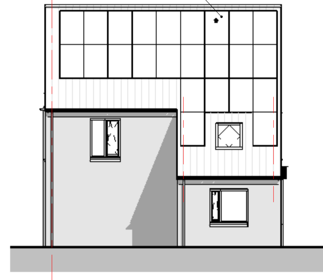
Linker zijgevel Blok A schaal 1:100
