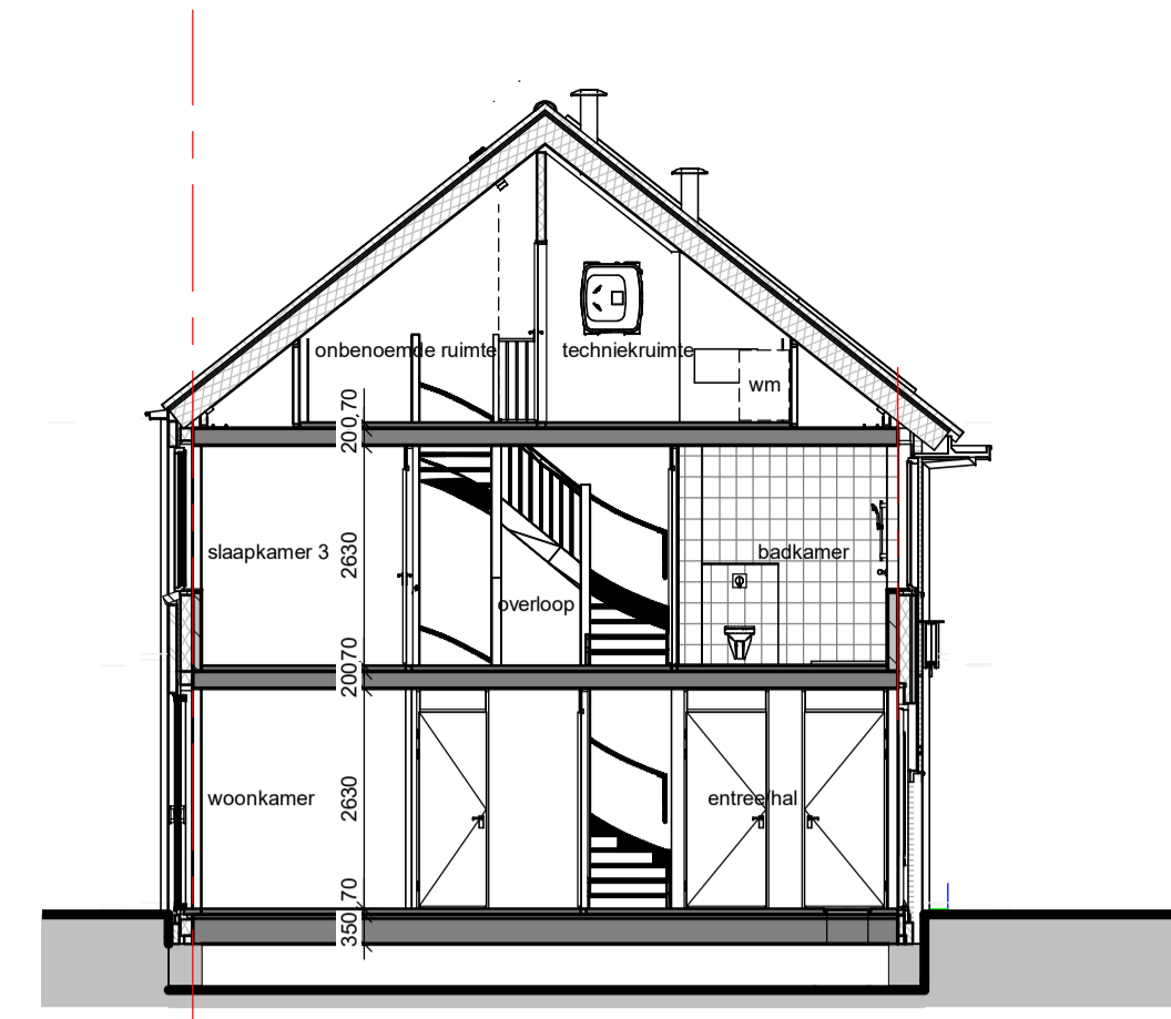
Doorsnede A-B schaal 1:100
