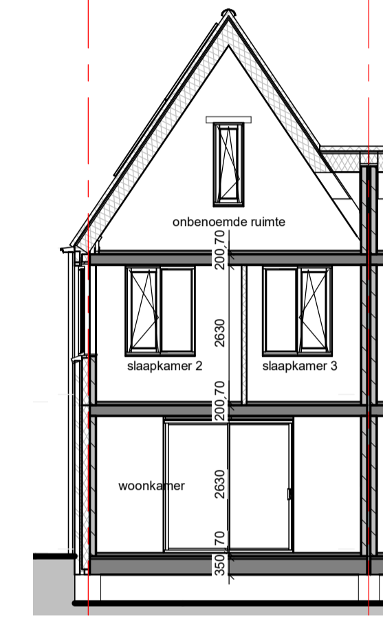
Doorsnede A-D schaal 1:100
