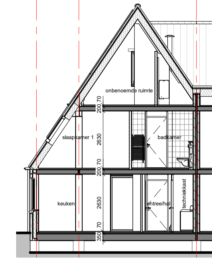
Doorsnede A-C schaal 1:100
