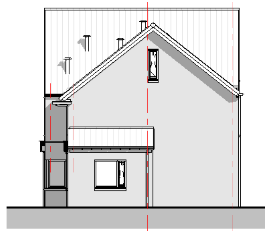
Rechter zijgevel Blok A schaal 1:100
