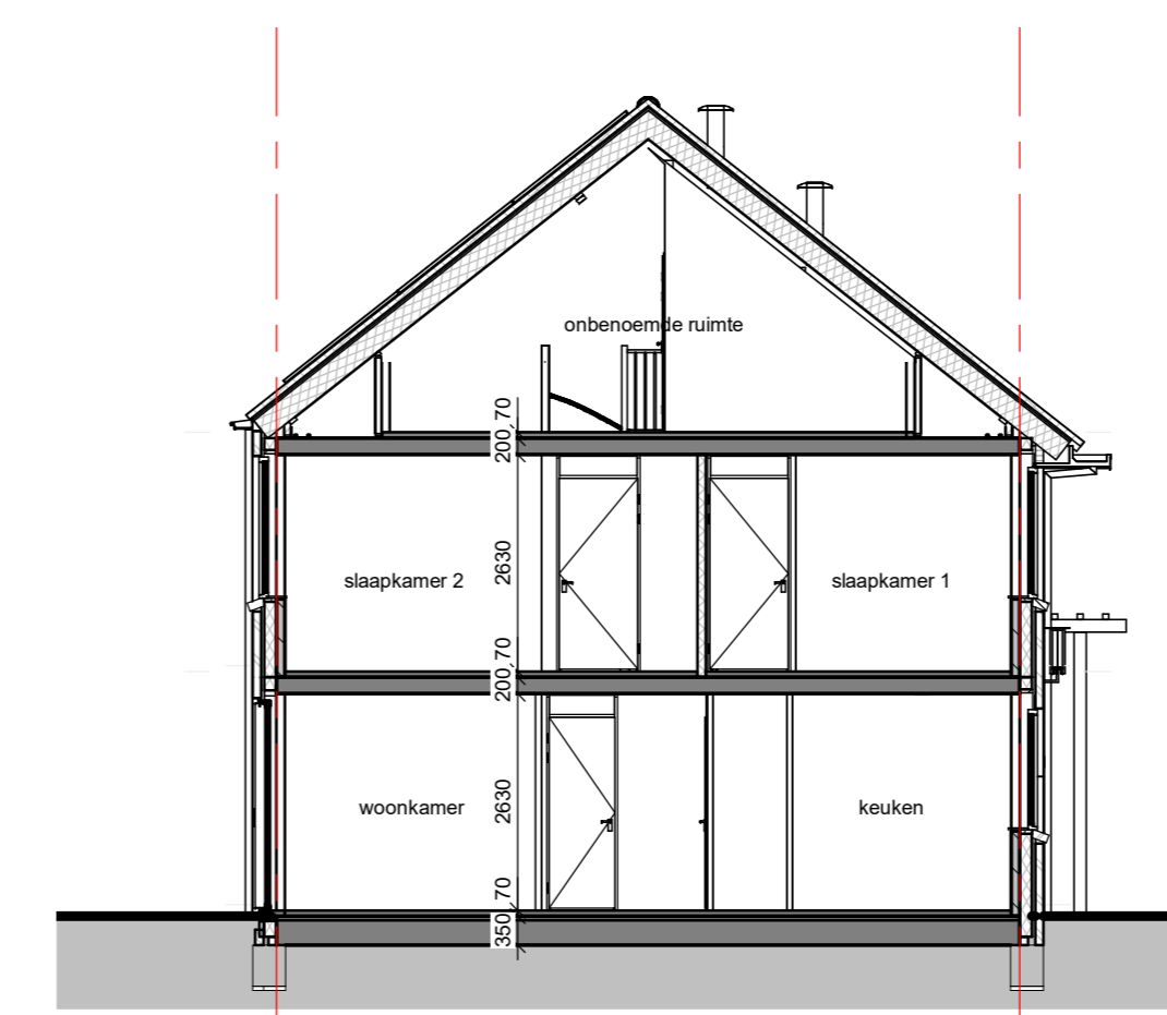
Doorsnede G-A schaal 1:100
