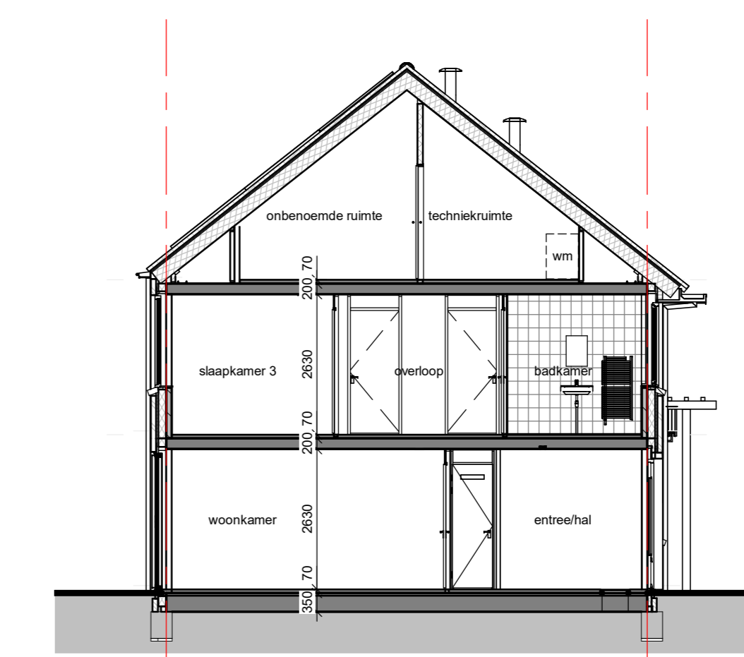
Doorsnede G-B schaal 1:100
