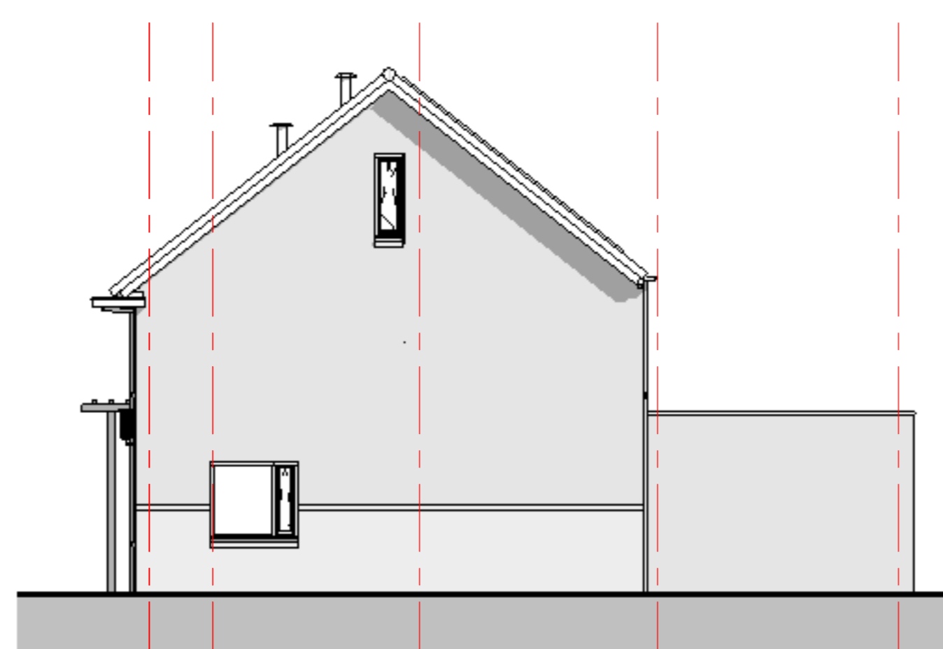
Rechter zijgevel Blok G schaal 1:100
