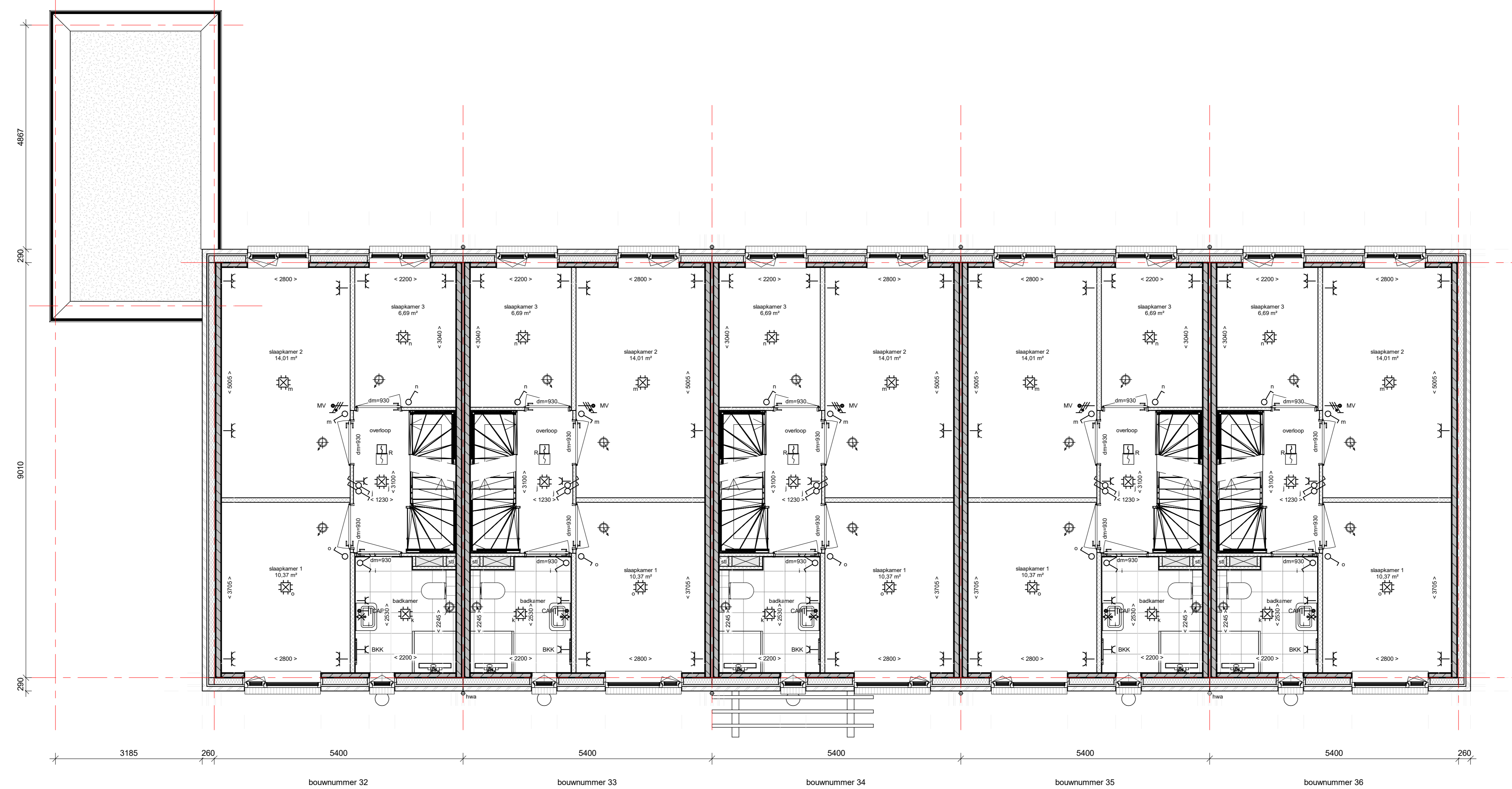
1e verdieping schaal 1:50
