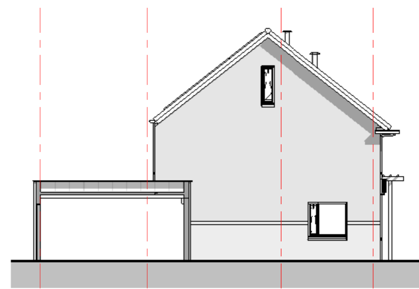
Linker zijgevel Blok G schaal 1:100
