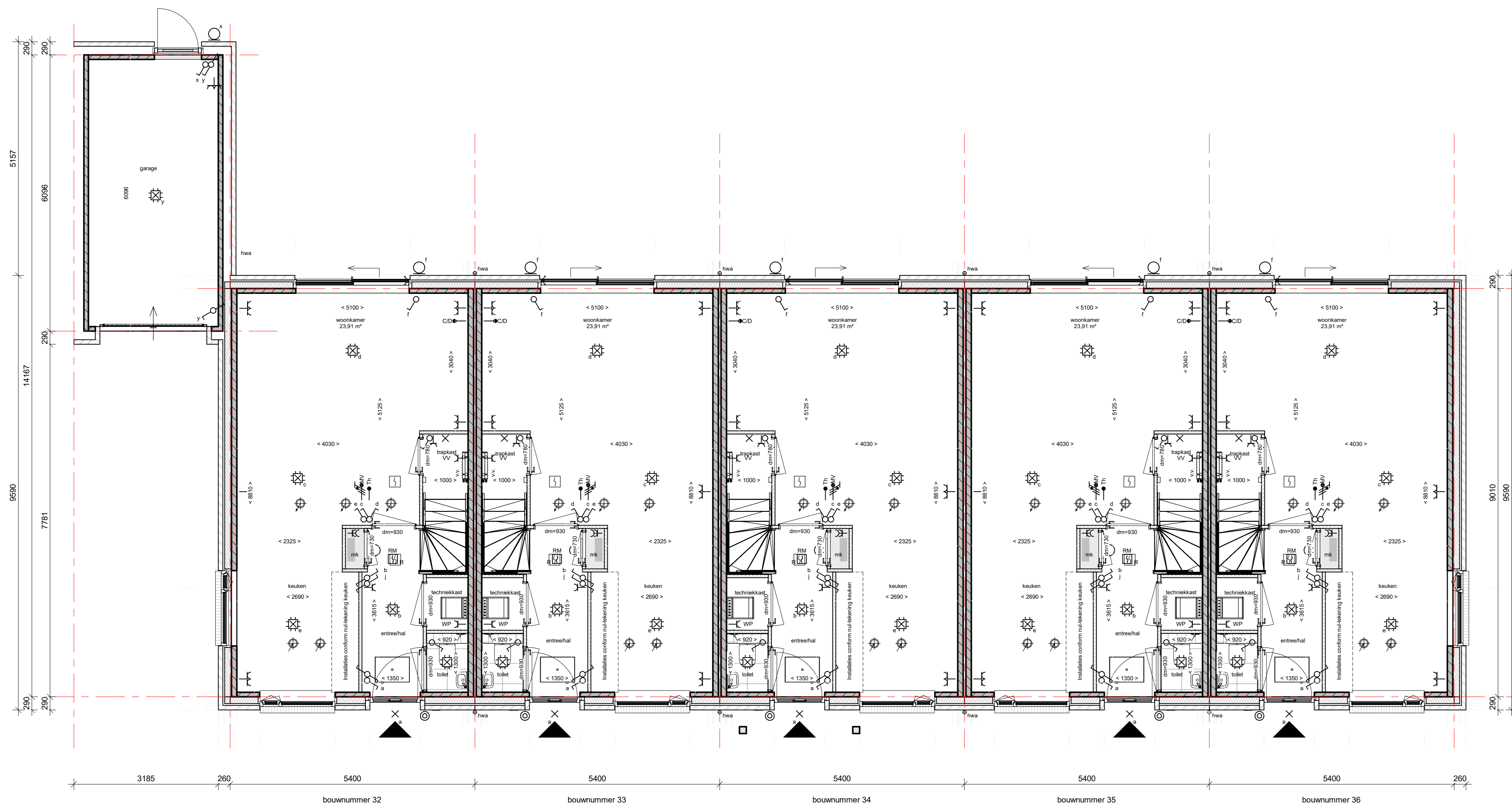
begane grond_Blok G schaal 1:50
