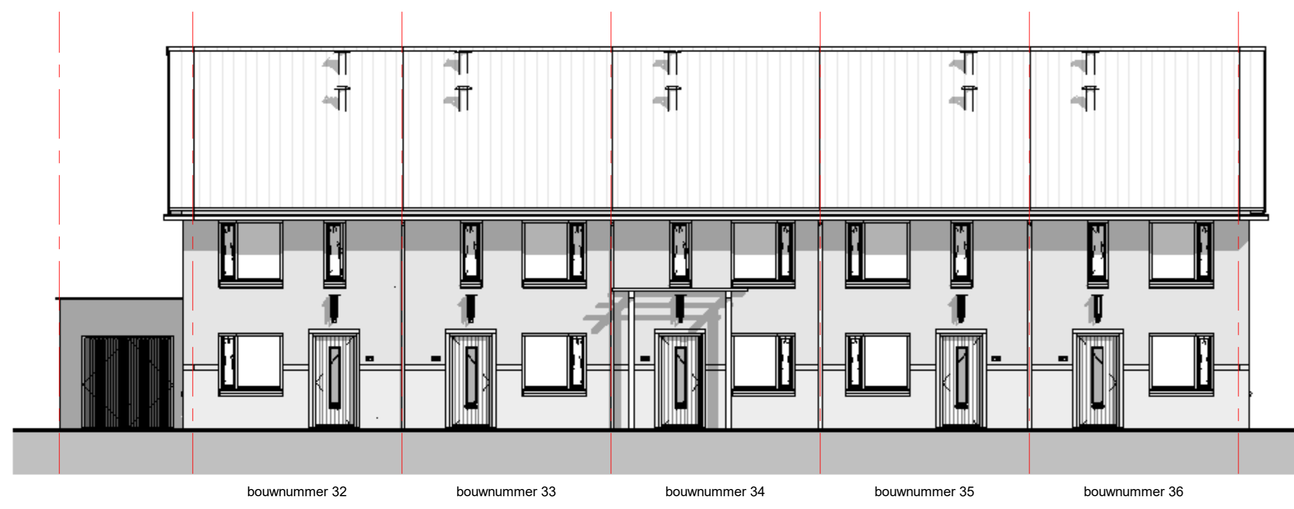
Voorgevel Blok G schaal 1:100
