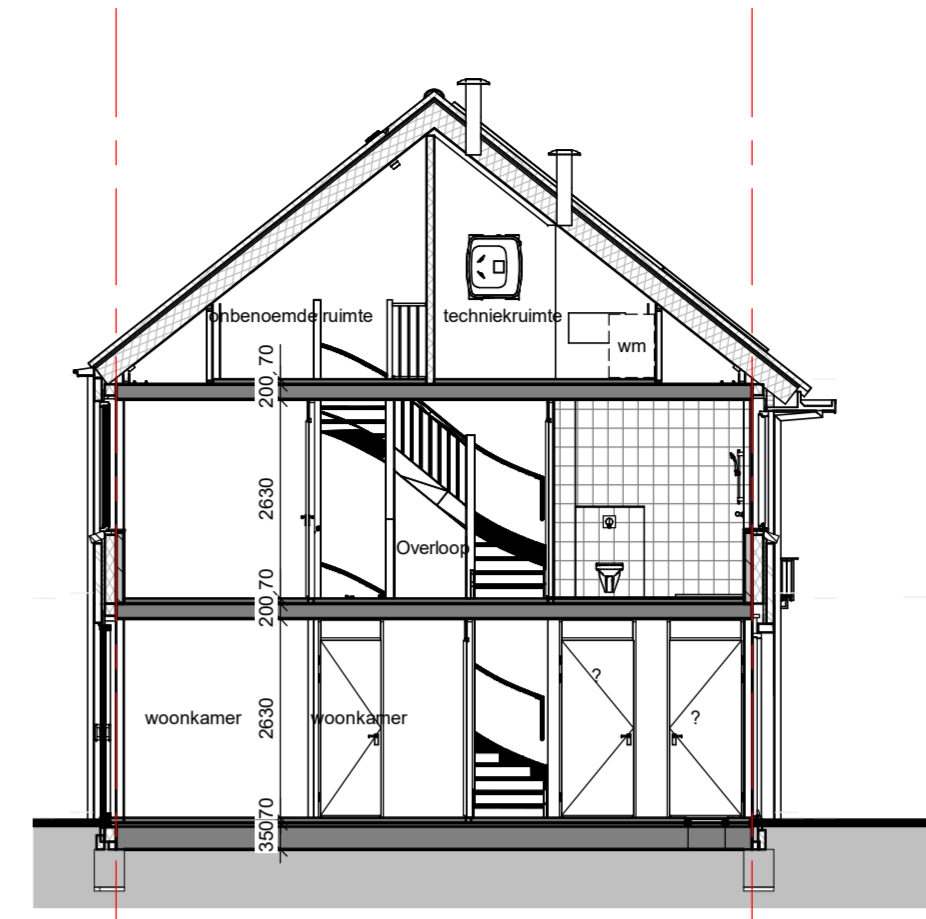
Doorsnede C-B schaal 1 : 100
