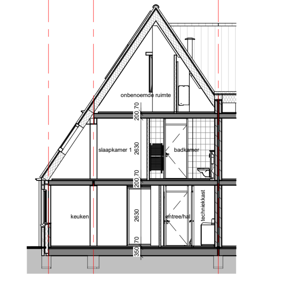
Doorsnede C-C schaal 1 : 100
