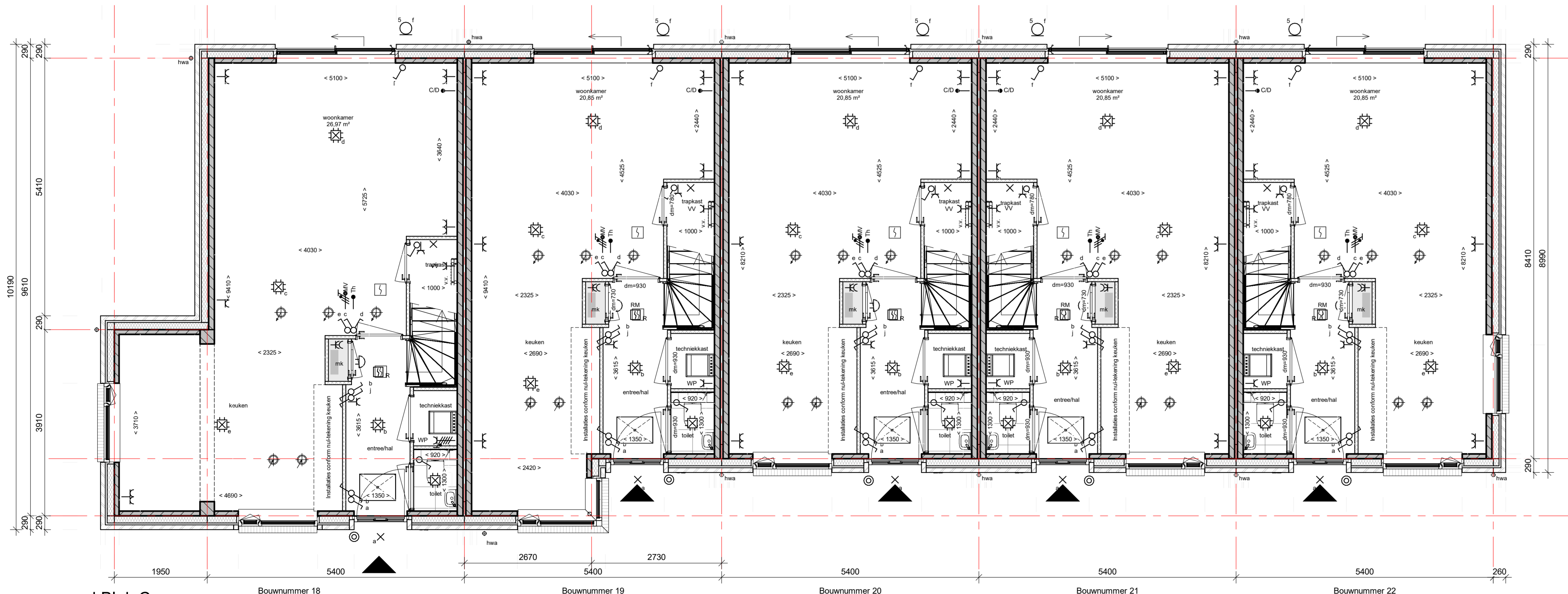
Begane grond Blok C schaal 1 : 50
