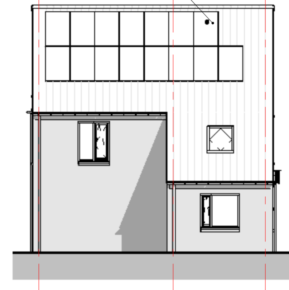
Linker zijgevel Blok C schaal 1 : 100
