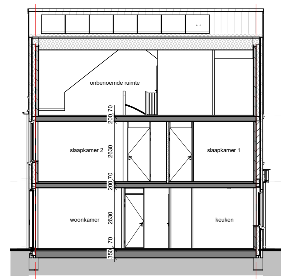
Doorsnede C-A schaal 1 : 100
