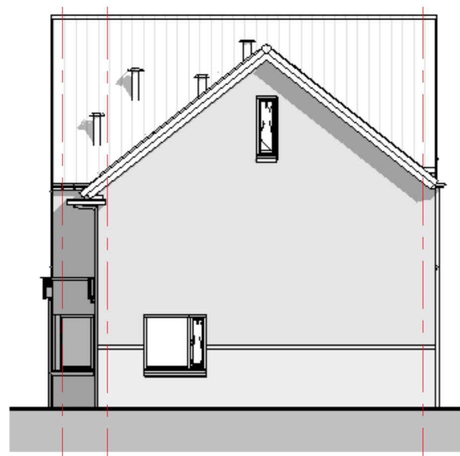
Rechter zijgevel Blok C schaal 1 : 100
