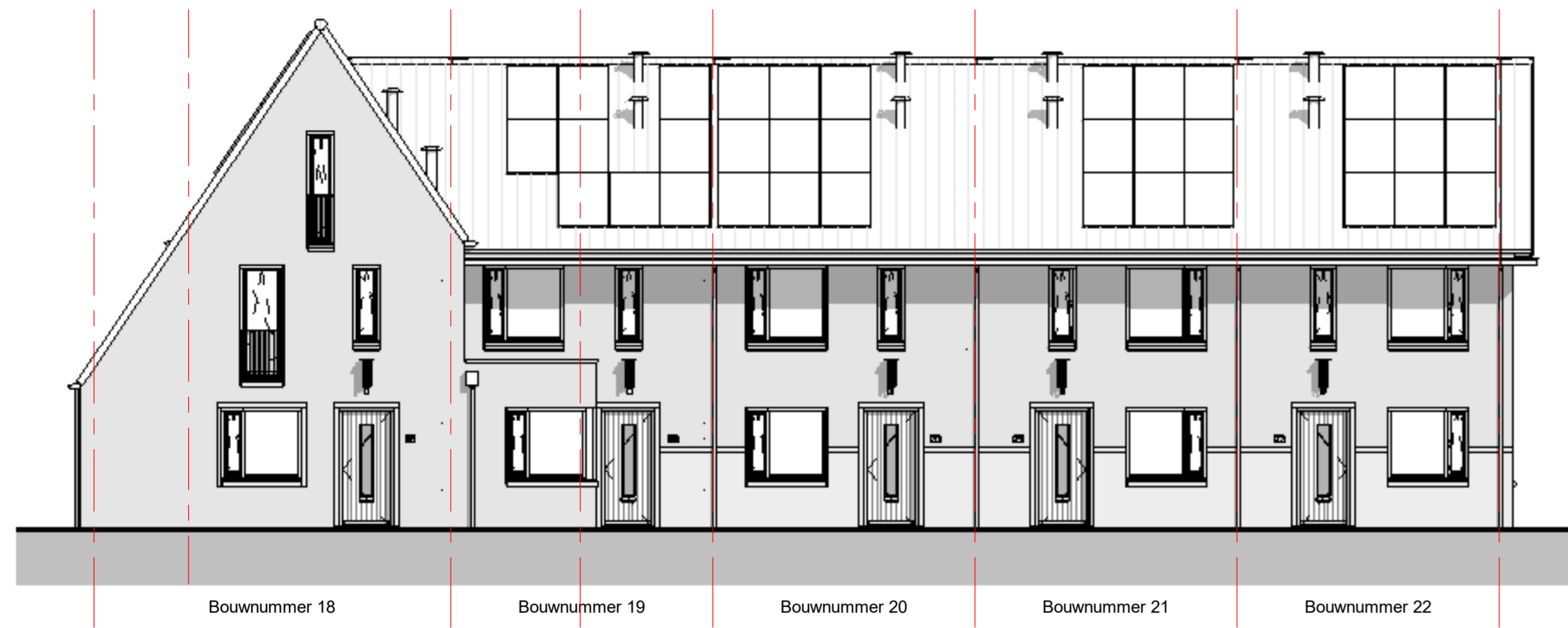
Voorgevel Blok C schaal 1 : 100
