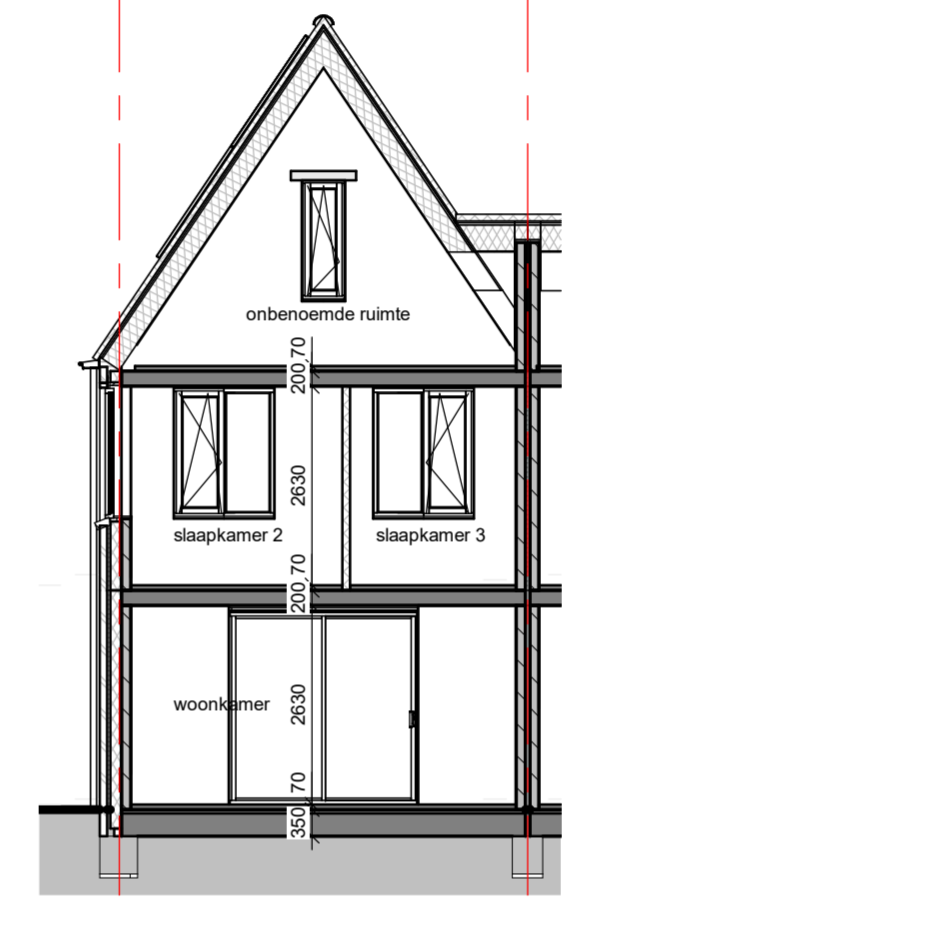
Doorsnede C-D schaal 1 : 100
