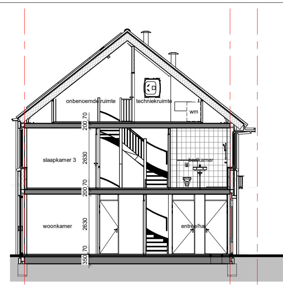
Doorsnede D-B
