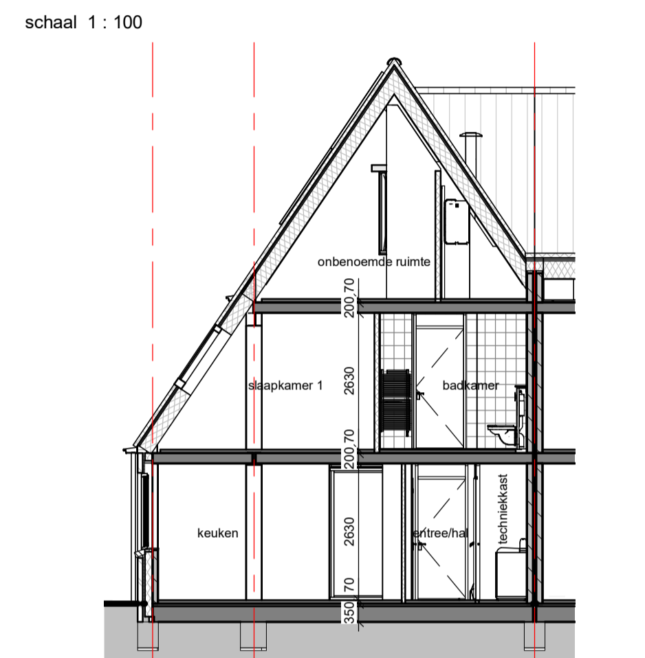
Doorsnede D-C
