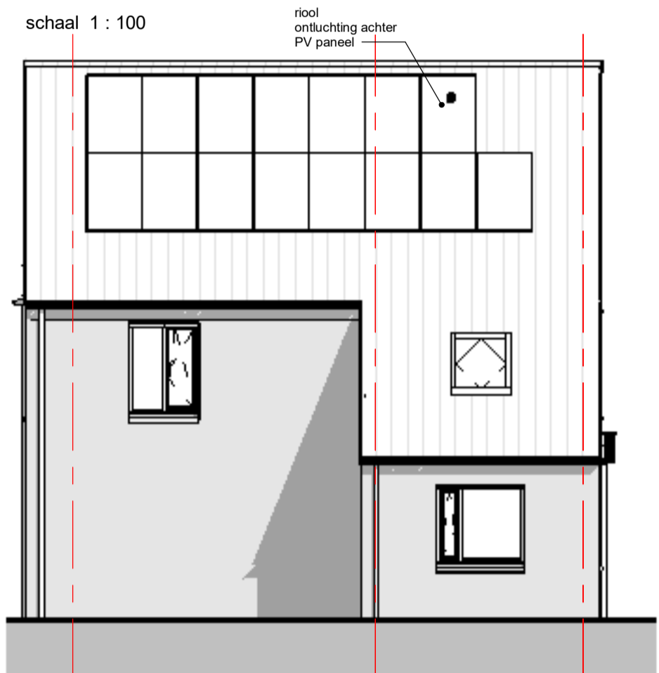
Linker zijgevel Blok D
