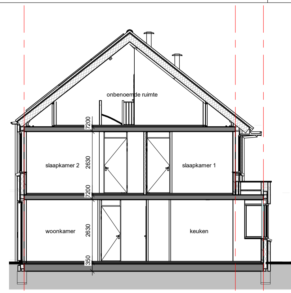
Doorsnede D-A
