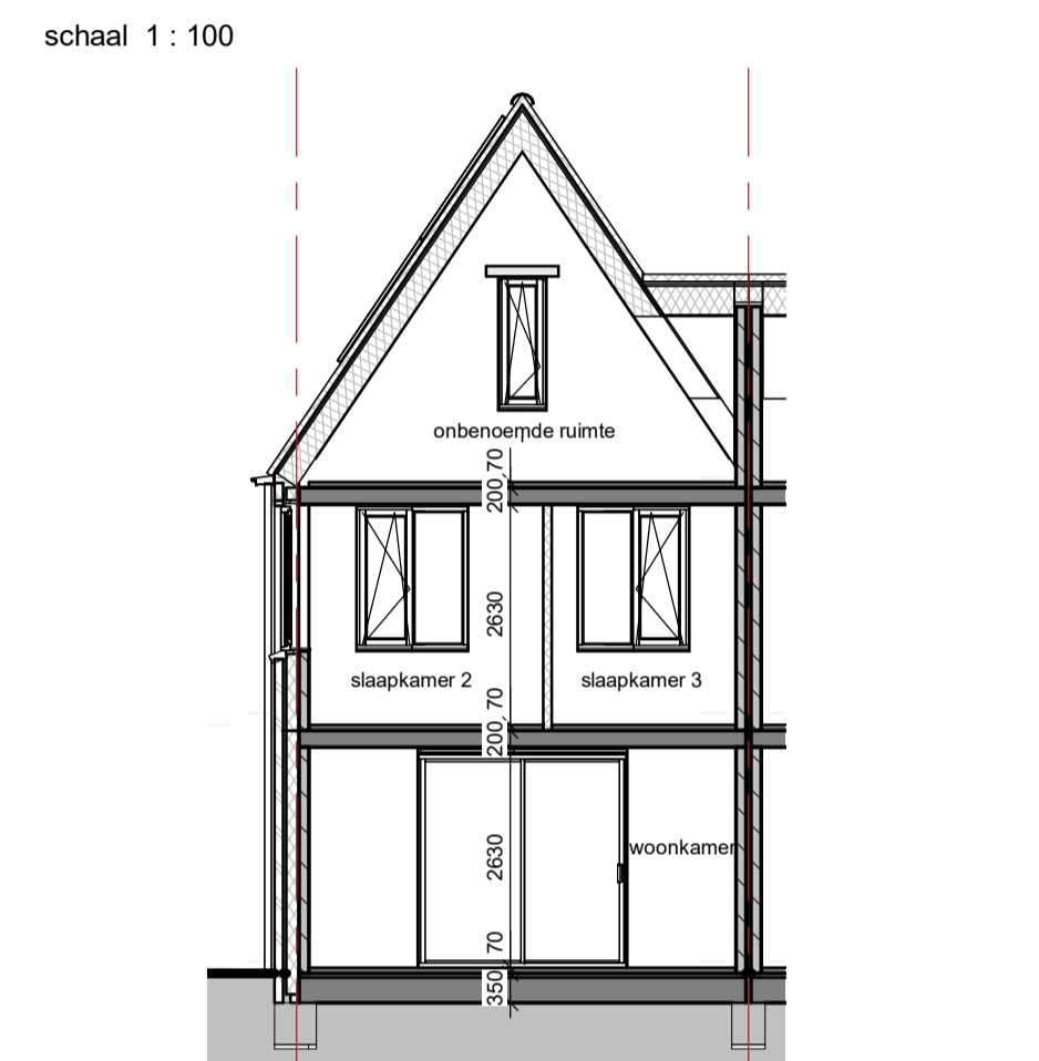
Doorsnede D-D
