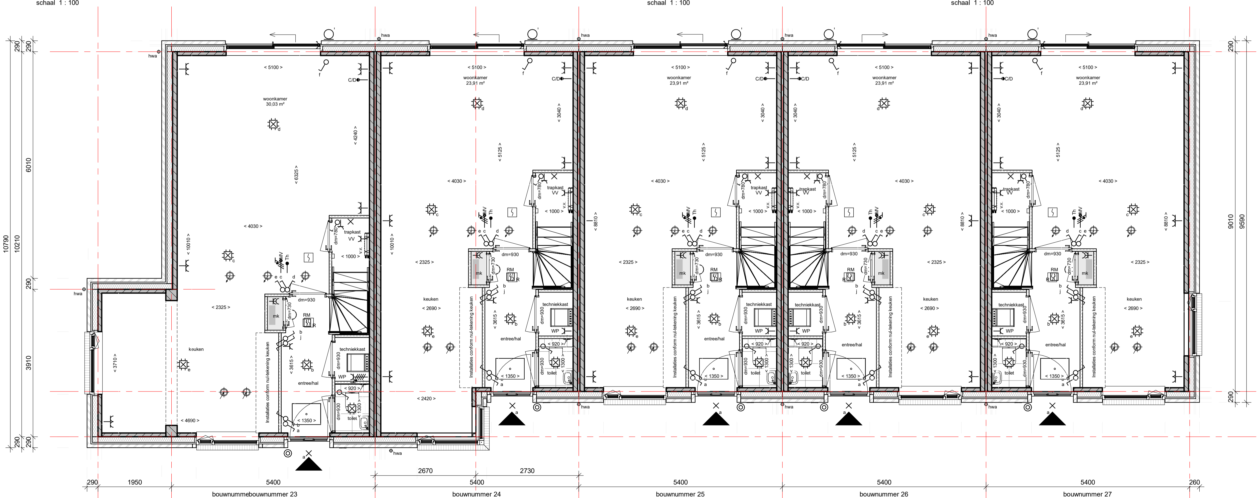
Begane grond Blok D
